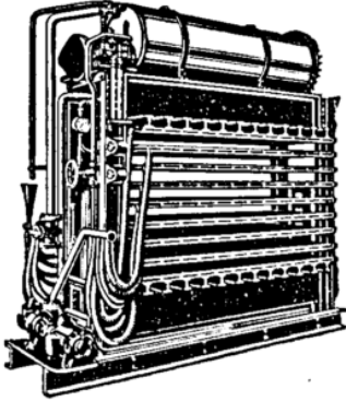
Hydr. Furnierschnellpressen mit Holz- und Kühlplatten
