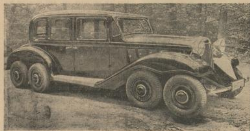
Das Auto mit 8 Rädern. Ein Berliner Konstrukteur hat diesen Achtradwalzen erbaute, der sich durch größere Sicherheit und Stoßfreiheit auszeichnet.
