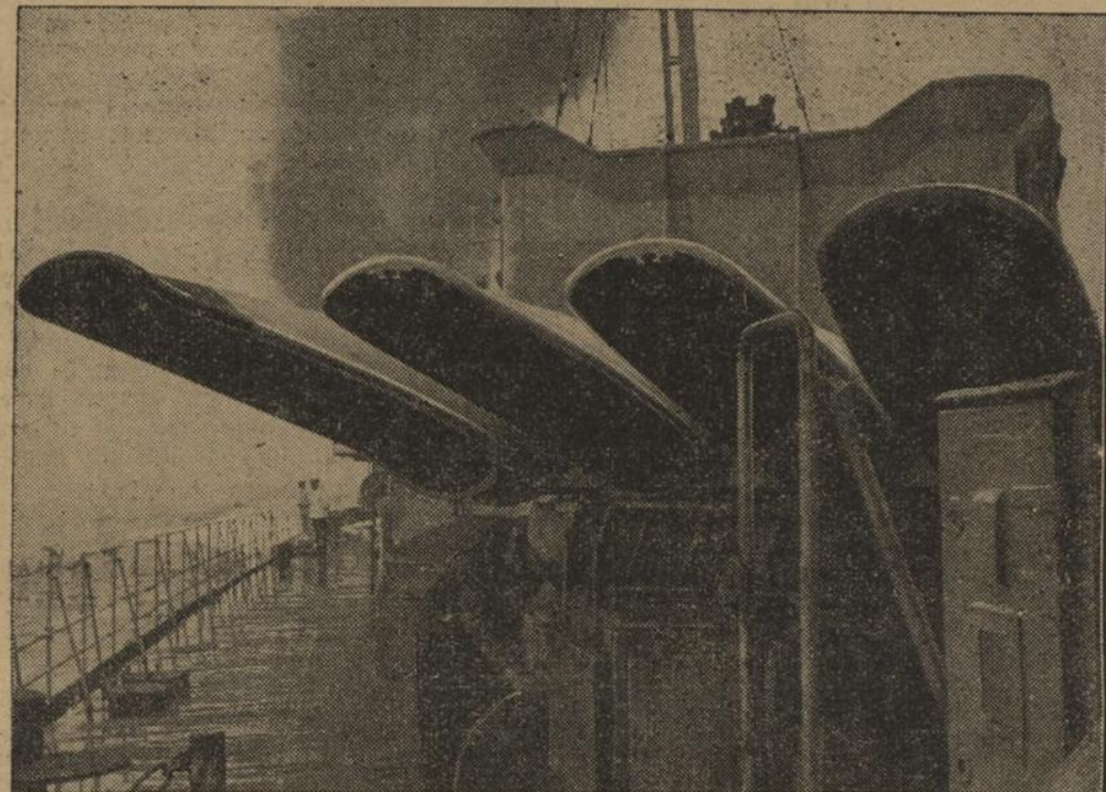
Torpedoschießen bei unseren Zerstörern. An-Bord des Zerstörers „Leberecht Maas“. Das Bild zeigt die wirkungsvolle Einstellung der riesigen Mündungen der Torpedorohre. (Scherl, Bilderdienst, M.)
