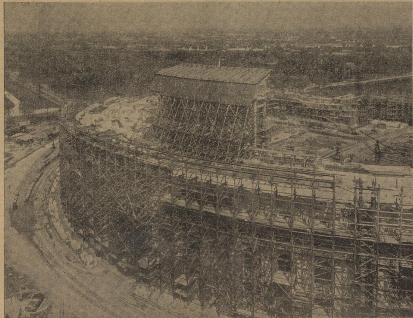
Das gigantische Rund der Kongreßhalle ist bis zur Höhe des Hauptgesimses eingerüstet. Der Scheitelpunkt des Daches wird mit 80 Meter fast die doppelte Höhe der heute aufgeführten Umfassungsmauer erreichen.
