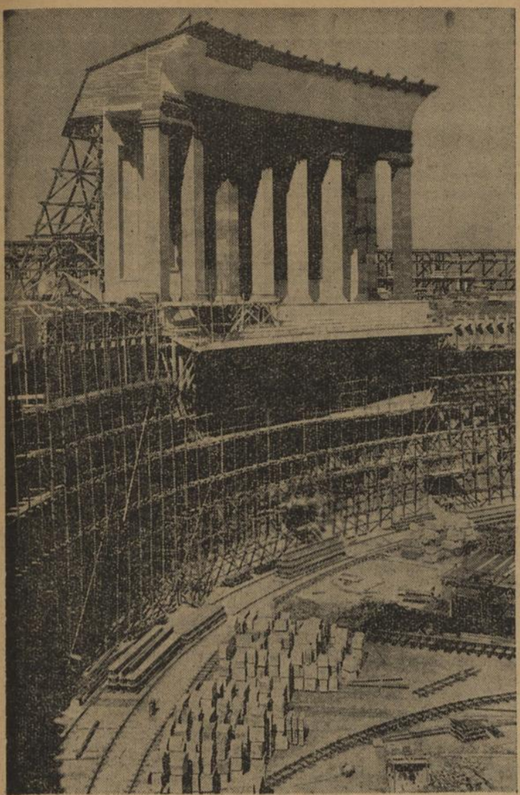
Blick in den Innenraum der Kongreßhalle, oben im Modell das von Granitsäulen getragene obere Gesims, auf dem das freitragende Dach aufgesetzt wird.
