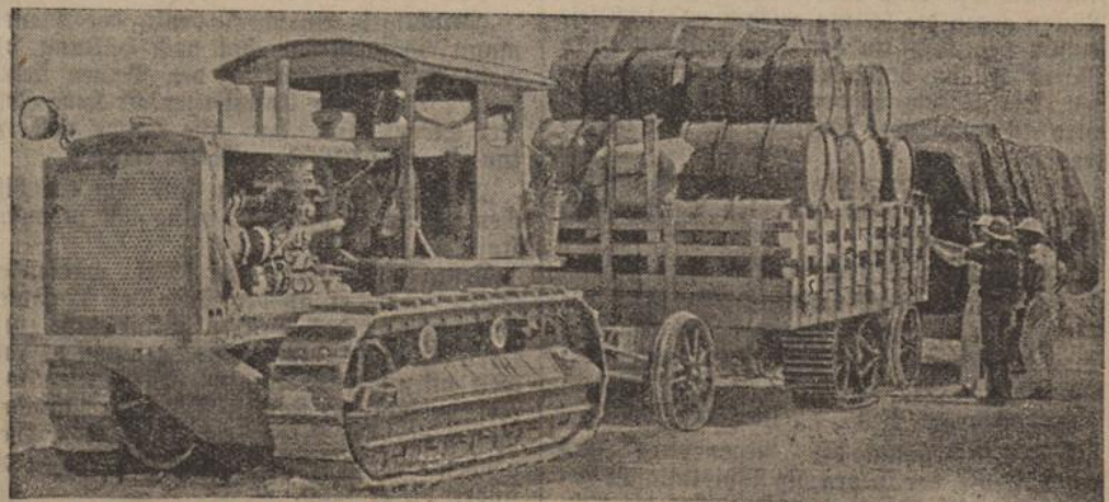
Lastwagen auf Raupenkette. Um der Schwierigkeiten, die das weglöse Gelände in Abessinien bietet, Herr zu werden haben die Italiener auch ihre Lastwagen mit Raupenkette ausgestattet, die von modernen Raupenschleppern gezogen werden. Mit ihnen werden Munition, Lebensmittel und Benzin an die Somalifront befördert. (Grafik-Bild-Zentrale, B.J.)
